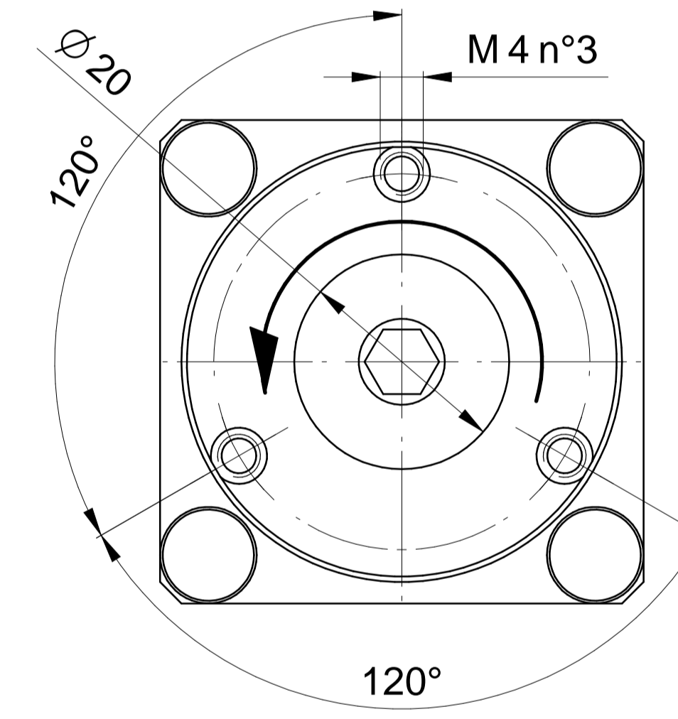
BLADE SPINDLE
