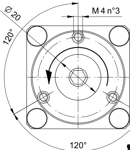
BLADE SPINDLE
