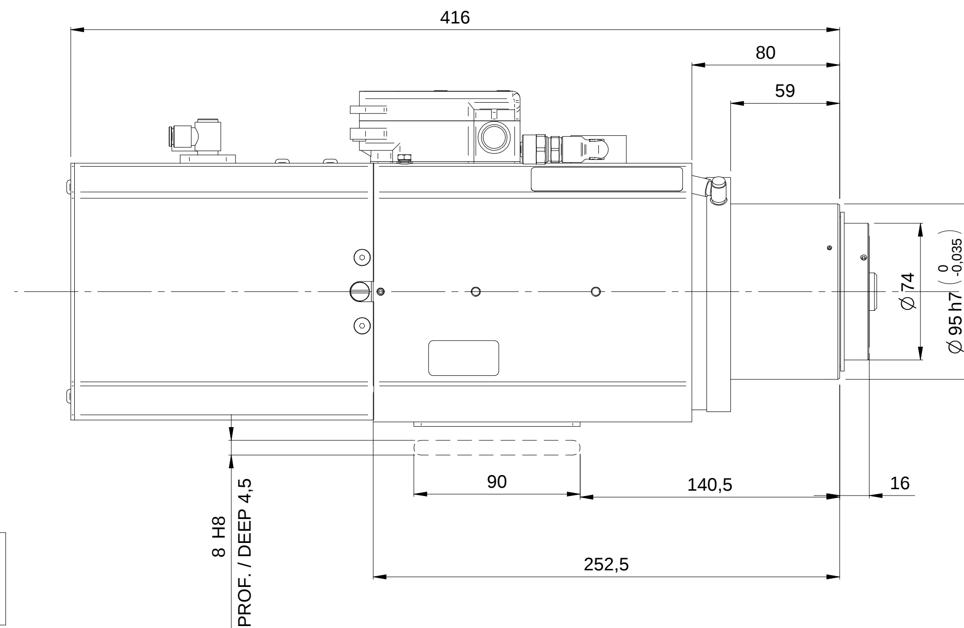
ATTACCO HSK 63F TOOL INTERFACE HSK 63F DIN 69893-6
