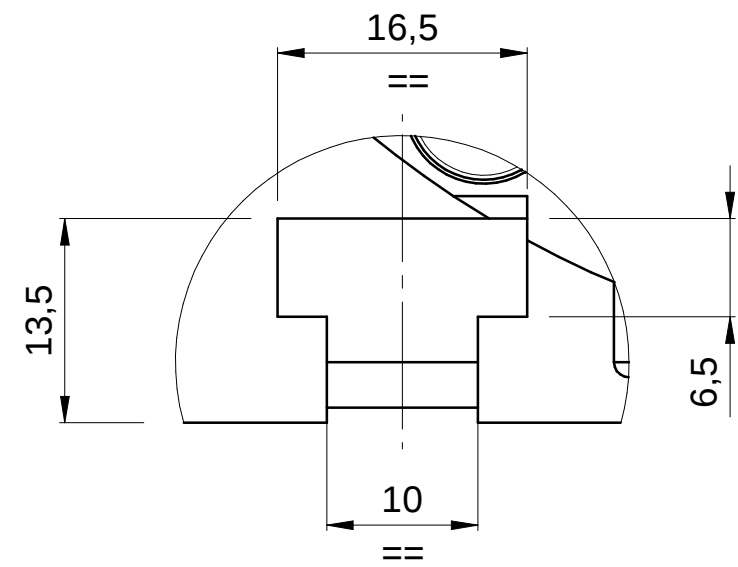
DETTAGLIO G
